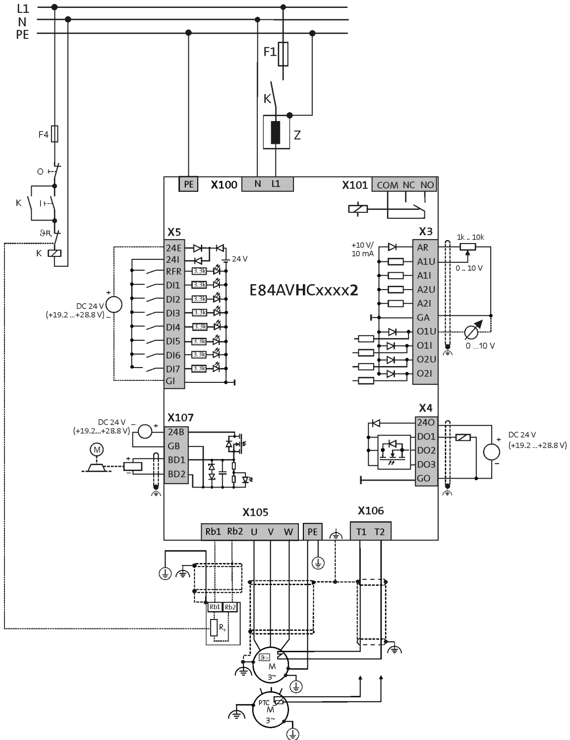
Verdrahtungsbeispiel Inverter Drives 8400 HighLine an 1 x 230 V
