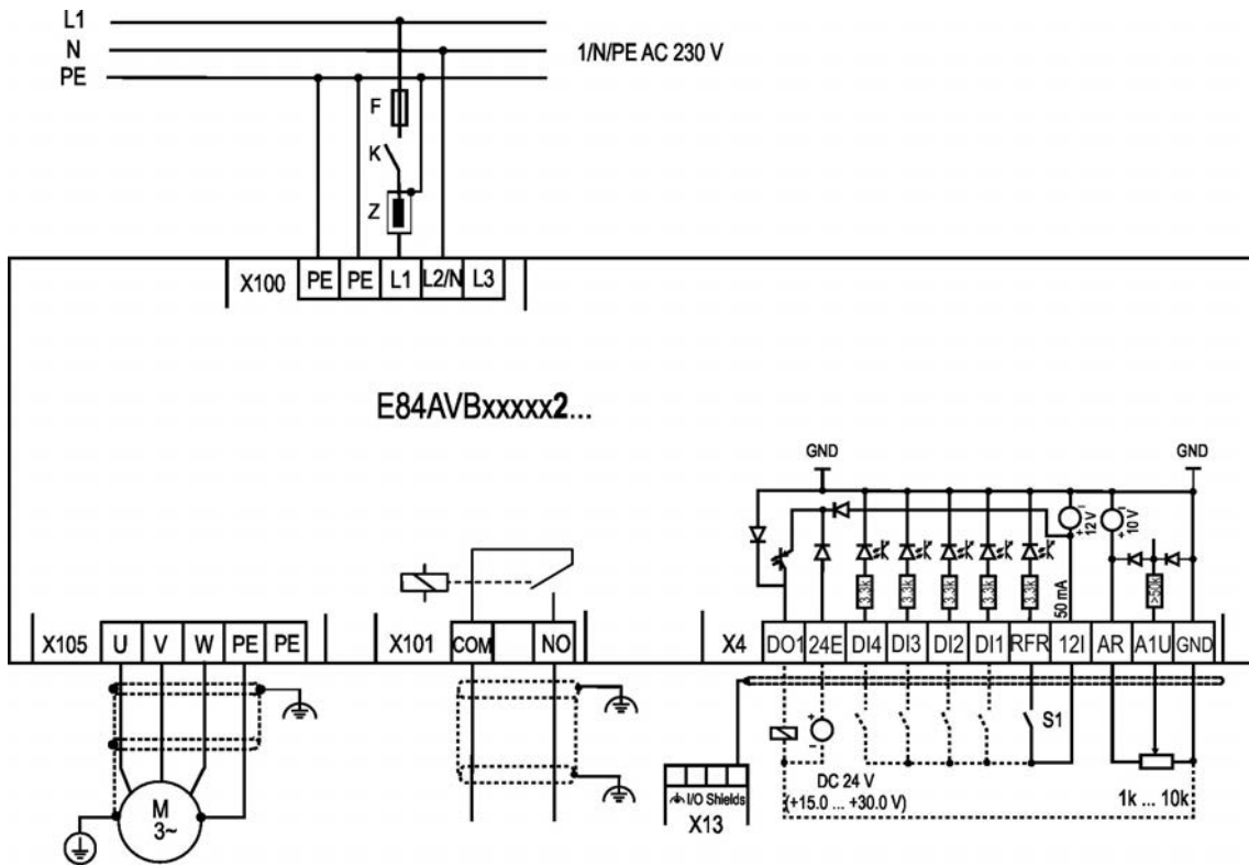
Verdrahtungsbeispiel Inverter Drives 8400 BaseLine (hier BaseLine D) an 1 x 230 V
